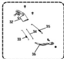
THROTTLE CONTROL ASSEMBLY ENSEMBLE DE COMMANDE D'ACCÉLÉRATEUR CONJUNTO DE CONTROL DEL ACELERADOR
