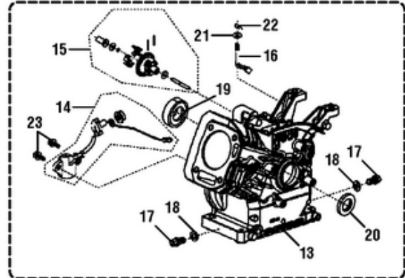
Crankcase Assembly Ensemble carter de vilebrequin Conjunto del cárter
