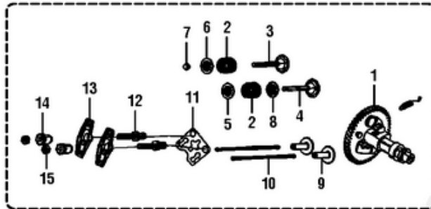
Camshaft Assembly Ensemble de l'arbre à cames Conjunto del árbol de levas
