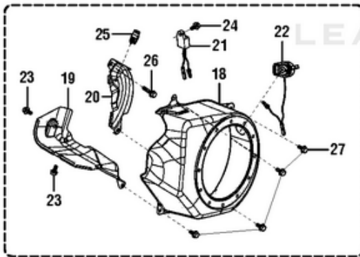
Lower Shroud Boîtier inférieure Cubierta inferior
