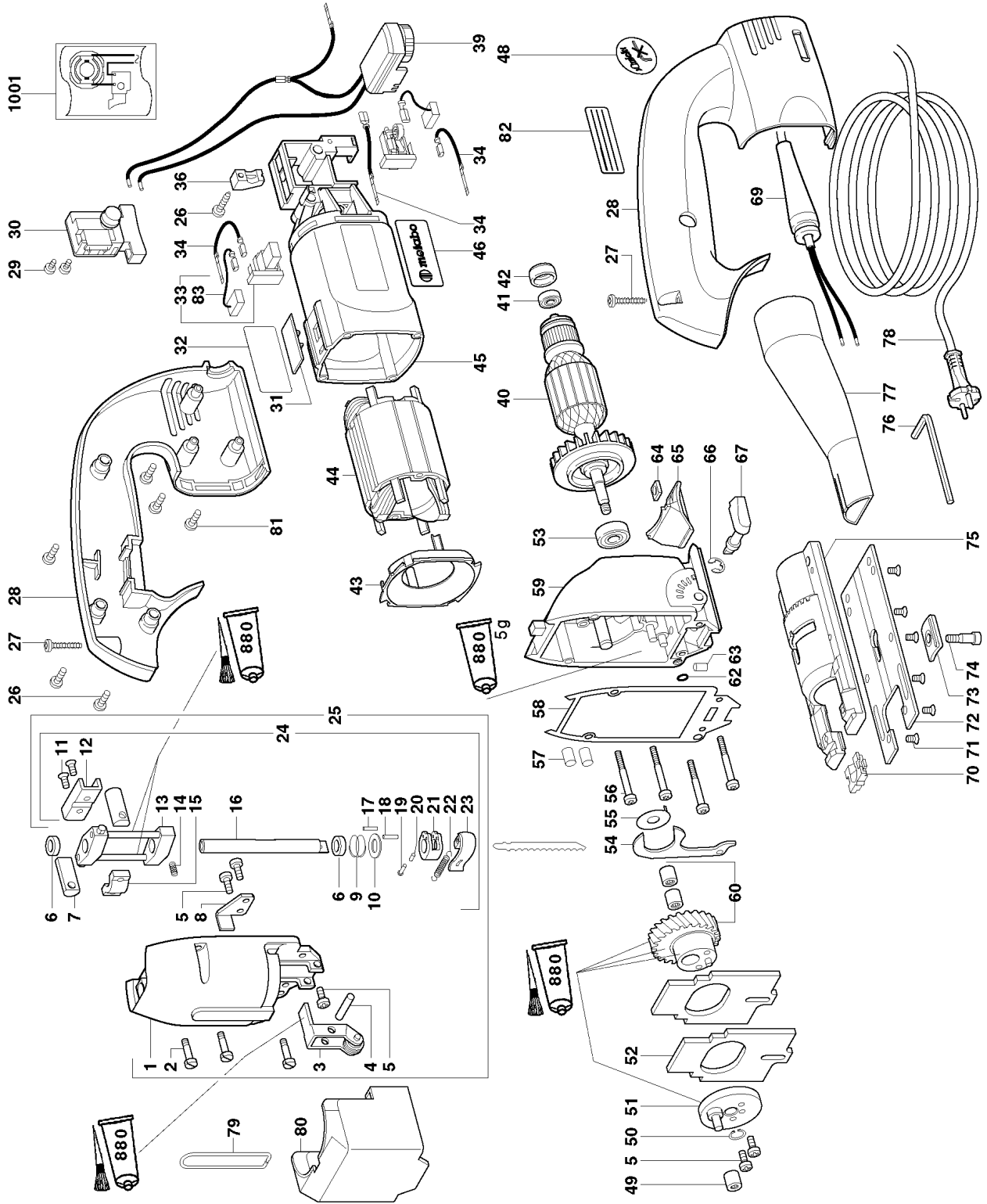
STEB 105 Plus 610600420
