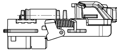
Stellrad vollst. / Selector wheel compl.
