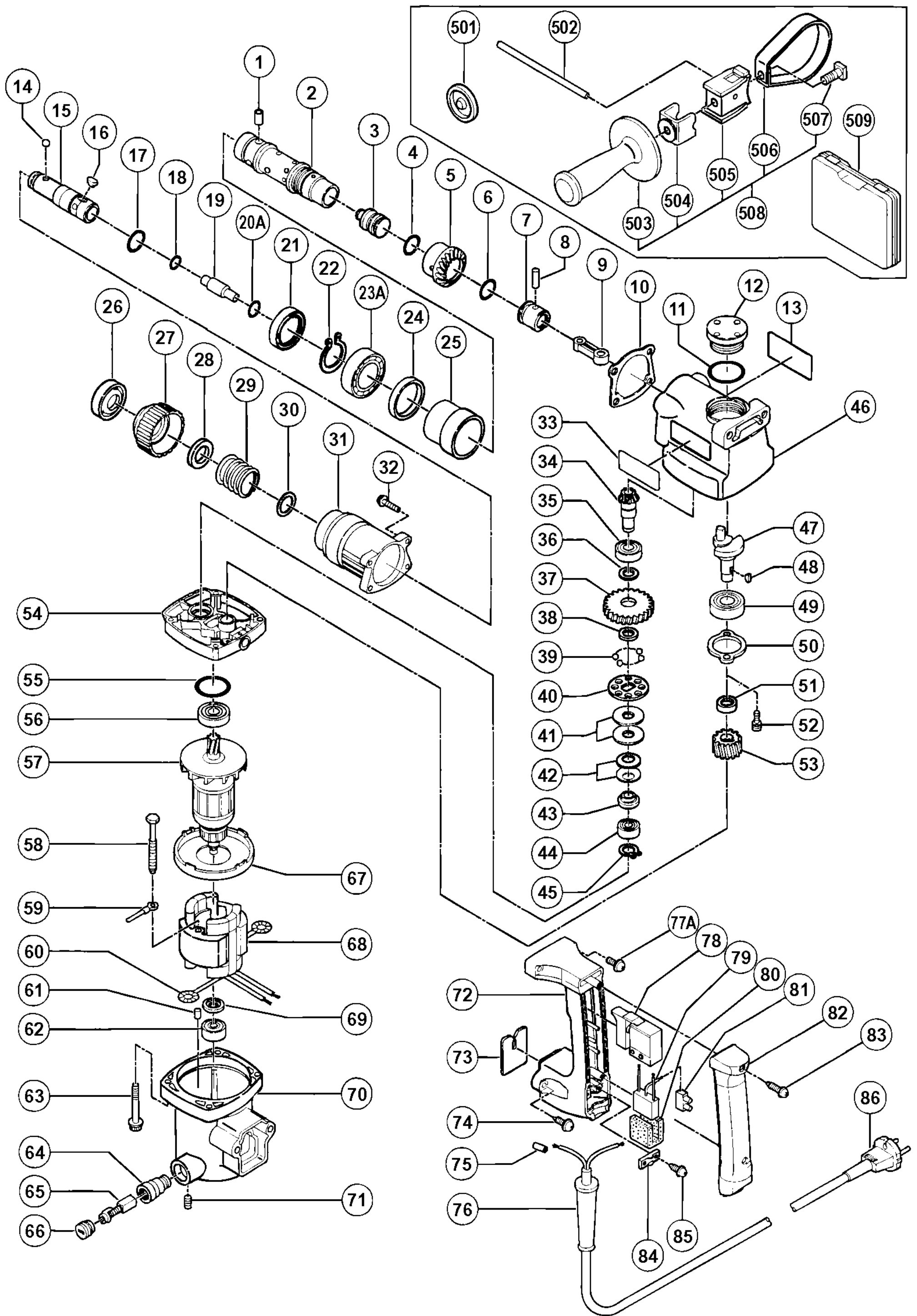
形 名 DH25PA
