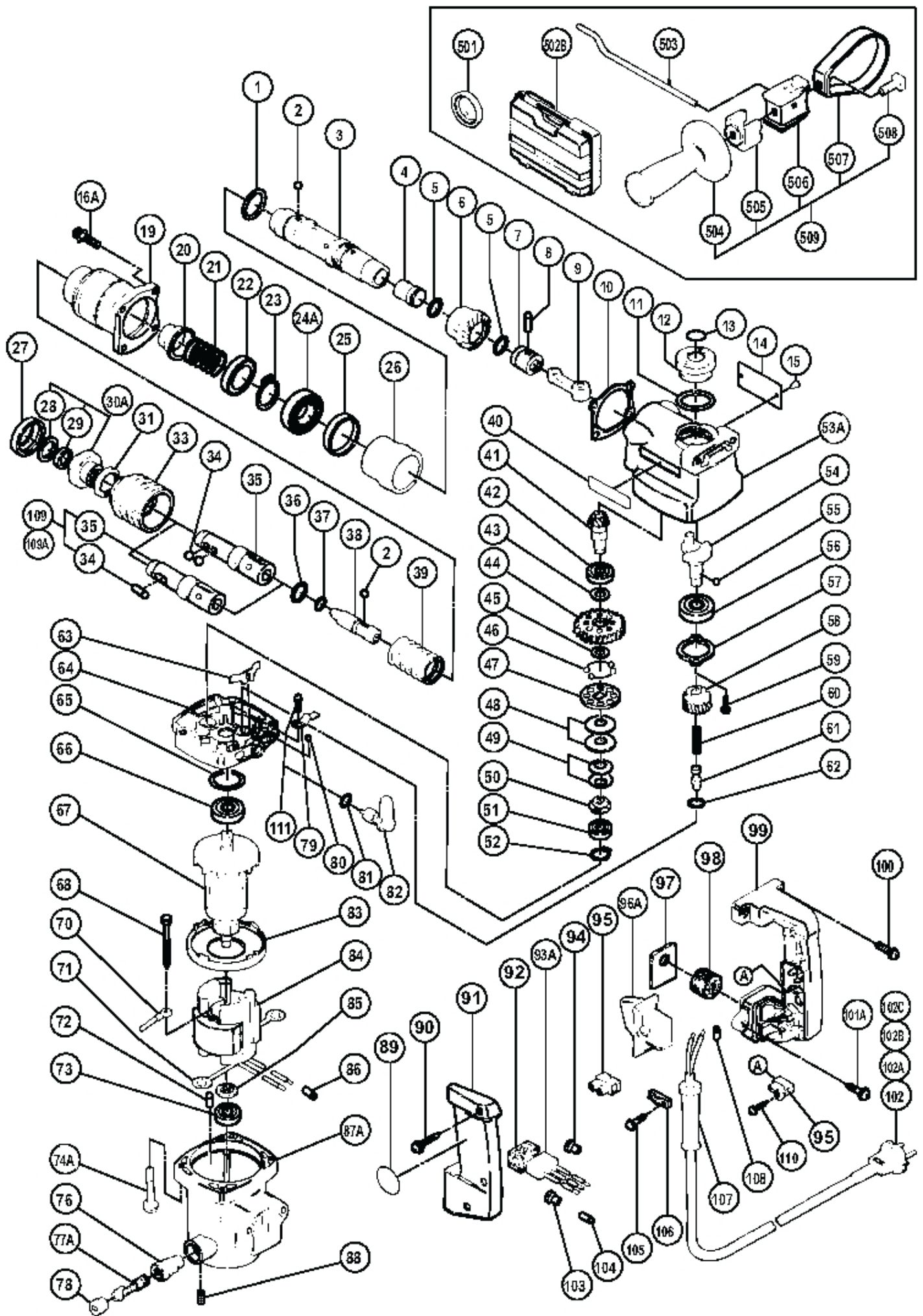
形名 DH20V
