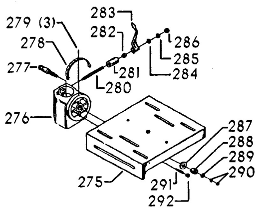
20-660 TILT TABLE
