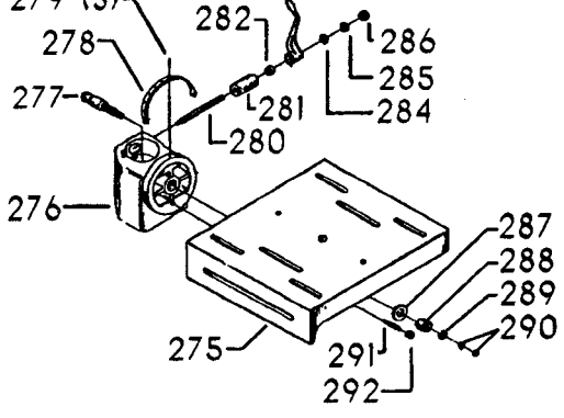
20-660 TILT TABLE
