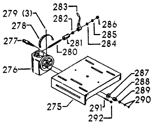
20-660 TILT TABLE
