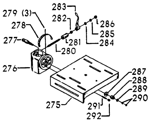
20-660 TILT TABLE
