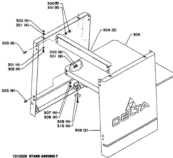
1313320 STAND ASSEMBLY
